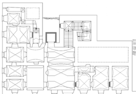
Skalka (okr. Litoměřice), plán přízemí zámku. Šedě značeny mladší konstrukce a zazdívky, čárkovaně obě tzv. skalní místnosti. Měřítko 25 metrů. Stav 16. července 1999, zaměření Jiří Peták starší a autor, kresba autor.
