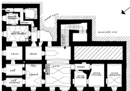
Skalka (okr. Litoměřice), plán přízemí zámku. Jeho autor zaznamenal celý rozsah podlaží včetně dvou tzv. skalních místností, později znepřístupněných. Nevypořádal se však s rozmístěním kleneb v jednotlivých prostorách, které jsou zjevně zaznamenány nepřesně. Stav v roce 1958, úprava autor.
